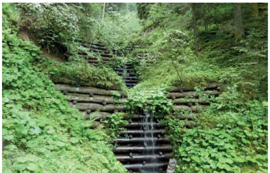
Regulierungsbauten müssen auf Zustand und Funktion kontrolliert werden.
