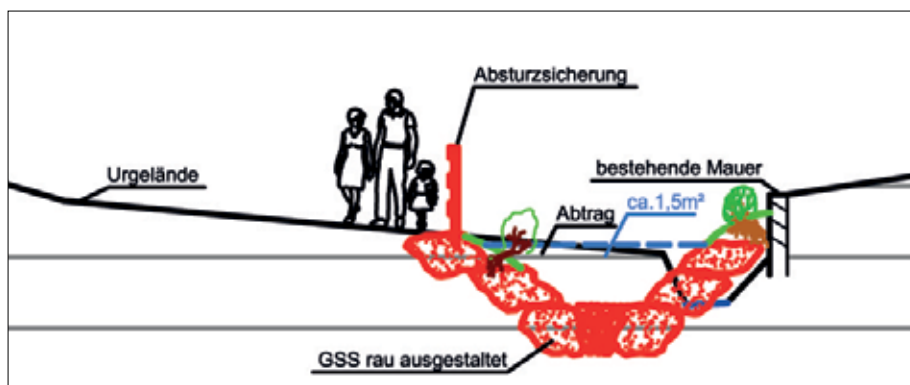
Querprofil der Ruifachbachl-Verbauung
