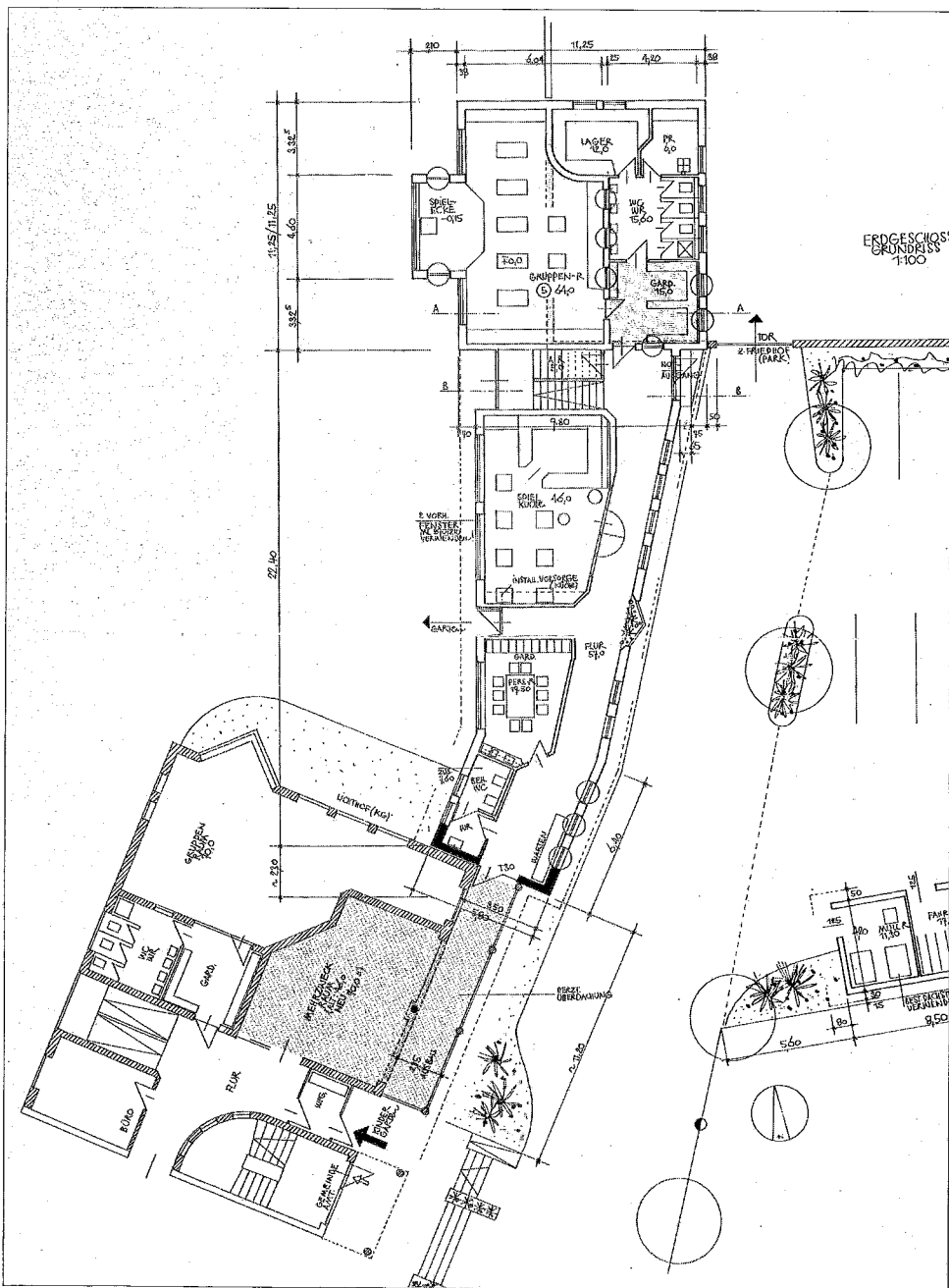
Erdgeschoßgrundriß des Kindergartenanbaues
