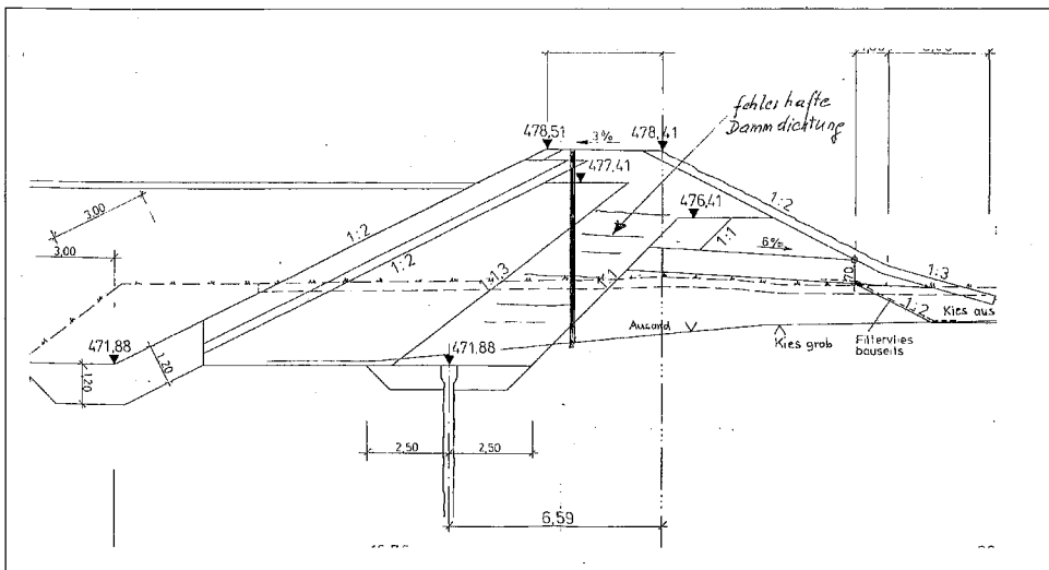
Schematische Darstellung des Dammschnittes
