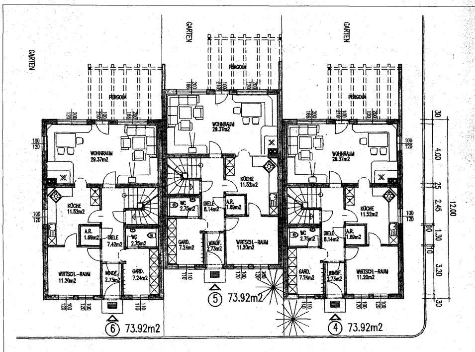
Erdgeschoßgrundriß (Muster, Einteilung individuell veränderbar)
