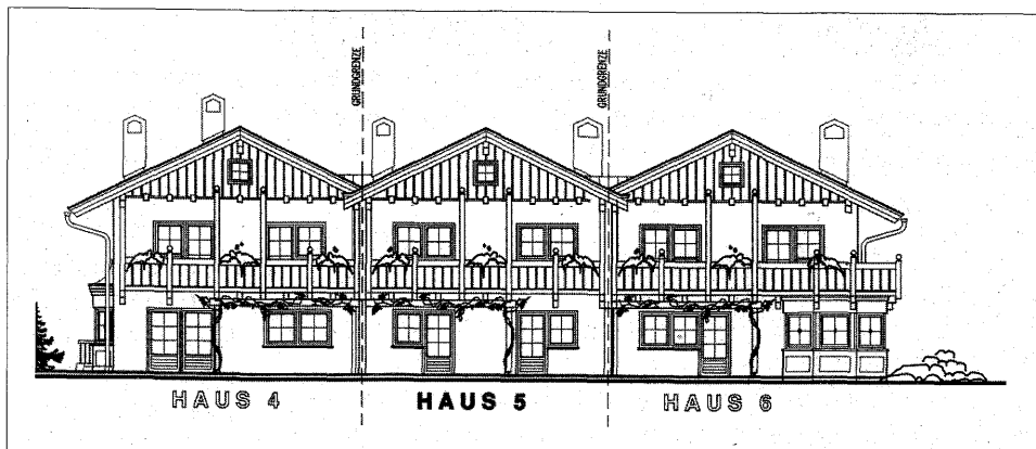
Südwestansicht
