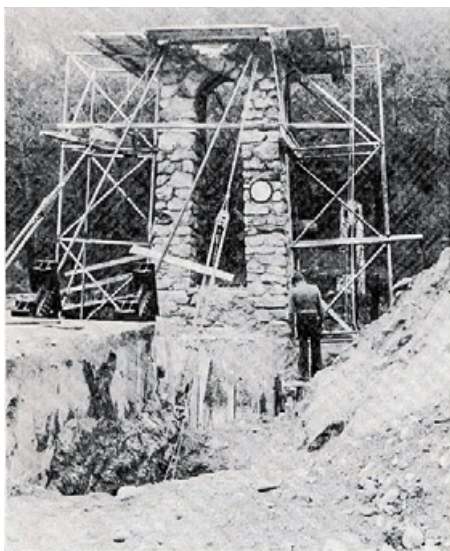
Die Stamser Hängebrücke erhält auf Grund des Autobahnbaues ein neues Fundament. Foto: Lechner
