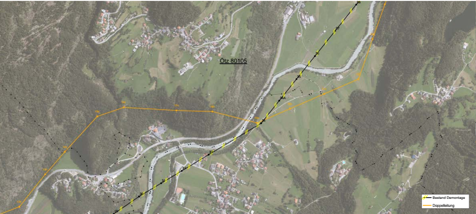
Leitungsverlauf Kändlschrofen bis Recyclinghof (Maststandorte sind mit Nummern bezeichnet)
