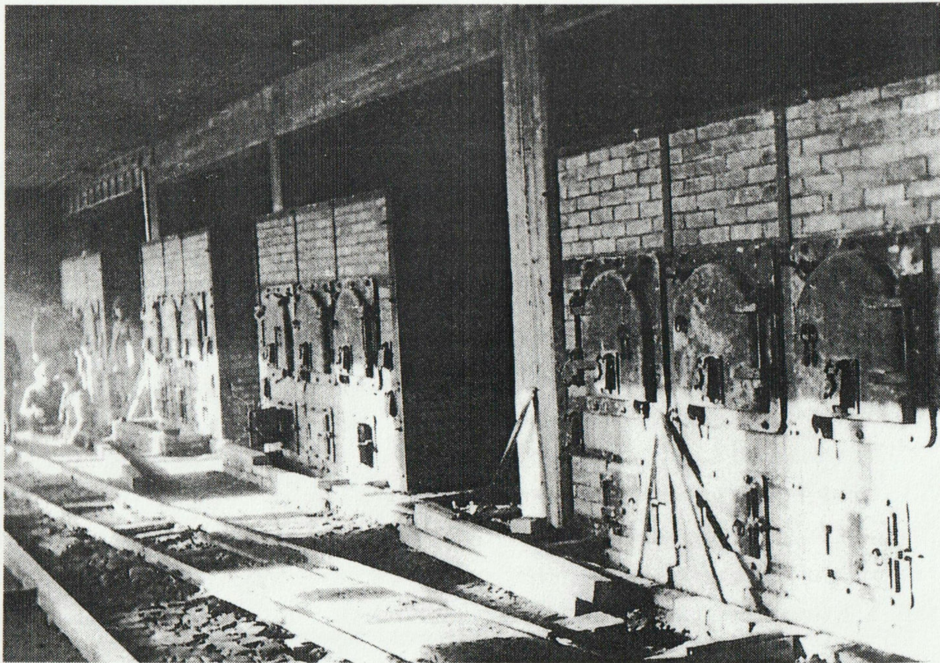
Deutscher Erfindergeist ersann maßgeschneiderte Lösungen für das KZ Auschwitz: Vier der fünf »Dreimuffelöfen« im Krematorium II.
