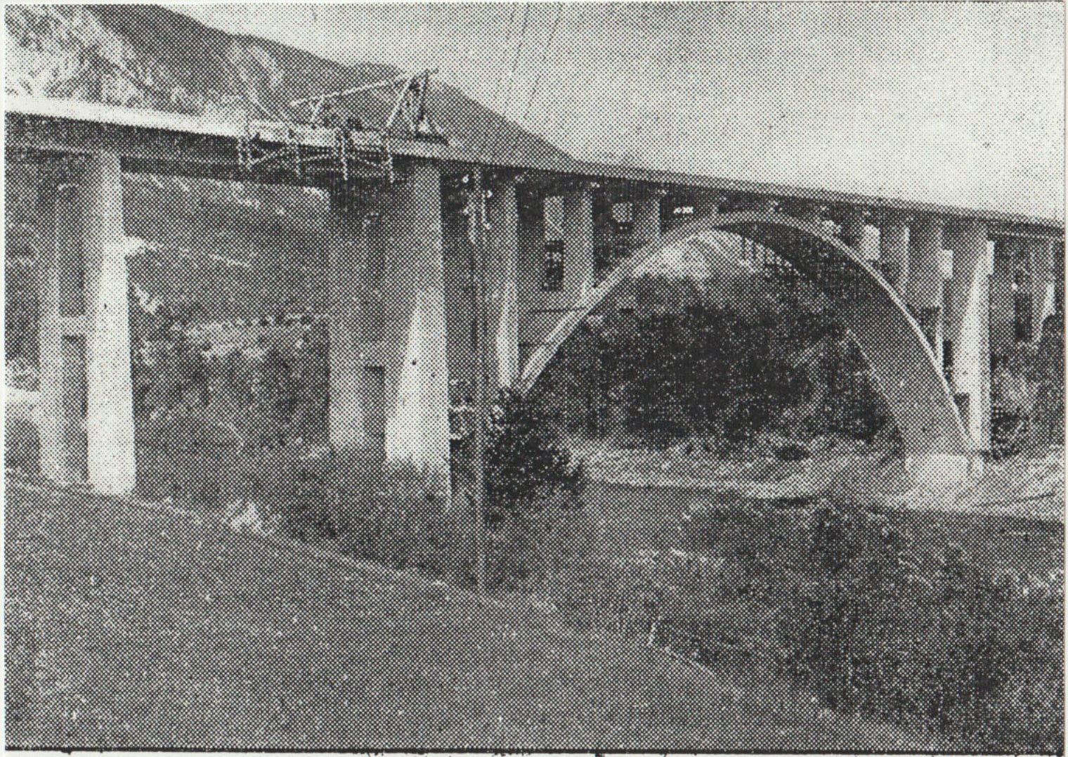
Die neue Reichsstraßen-Innbrücke, die gewaltigste Betonbogenbrücke Tirols
