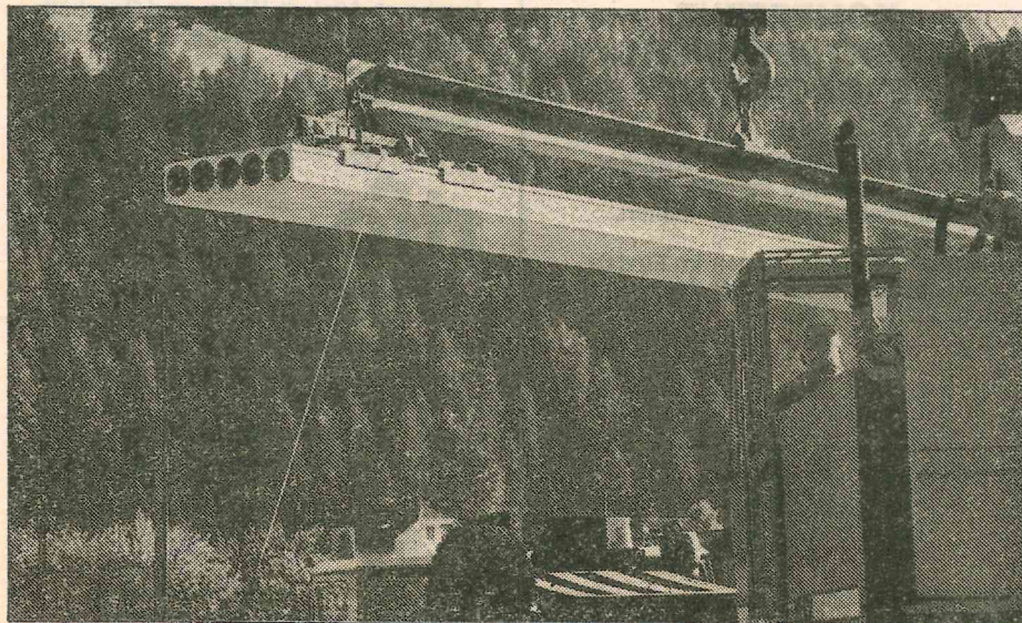
So sieht sie aus, die neue VS-Spannbeton-Hohldiele, hier bei der Montage.
