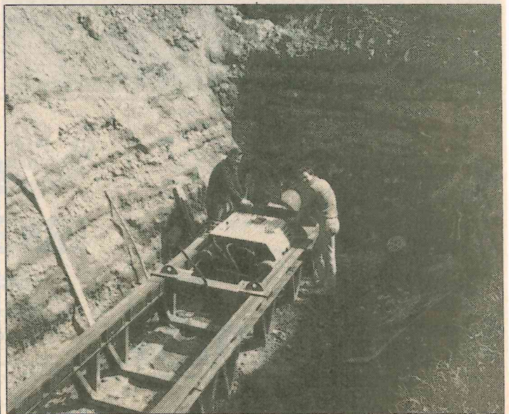
Im Bild die Pressarbeiten für den Kanal in Schlitters im Zillertal, Länge 40m, Rohrdurchmesser 50 cm.
