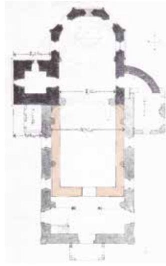
Grundriss der St. Notburga-Kirche in Eben: Dunkelgrau - Grundmauern der alten u. auch der neuen Kirche; Hellgrau - der barocke Anbau des Langhauses; Farblich - das gotische Langhaus, 1736 abgerissen
