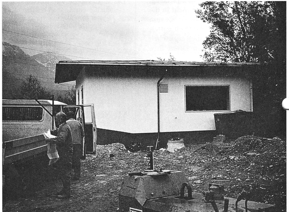
Zügig voran schreiten die Kanalbauarbeiten im Bereich Werth. Das neue Pumphaus (Bild) ist fast fertig gestellt, ebenso wie das neue Regenüberlaufbecken.
