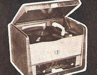
EUMIG Phono-Eumigette S 1799. — Der beliebte 7-Röhren-UKW-Druck- tasten-Super „Eumigette“ wurde durch ein 4-Geschwindigkeiten-Laufwerk er- weitert. Maße: 420 x 286 x 297 mm
