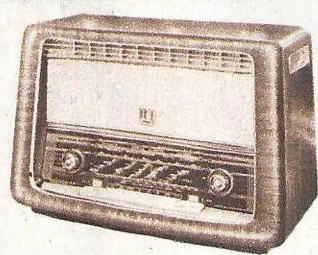
HORNYPHON Souverän S 3580. — 10-Röhren-Luxussuper mit vollendeter Tonwiedergabe durch Gegentakt- stufe, 2 Hochimpedanz-Lautsprecher, Höhenrundstrahltechnik. Maße: 660 x 455 x 305 mm
