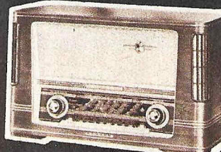
INGELEN Fidelio Luxus-Super 3 D „Das Konzertgerät von Rang“ S 3290.— 3D-Klangwiedergabe, 5fach-Klangabu- lator, 3 Sender-Soforteinstellung. Maße: 610 x 385 x 245 mm
