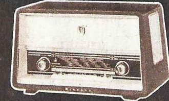
MINERVA Tempocord S 2520.— 8-Röhren-Großsuper mit Drucktastenbereichswahl und Drucktastensklangregister. Duplextrieb, Ferritantenne. Maße: 550 x 320 x 250 mm
