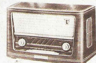
RADIONE Duplex Register 58 S 2370.— Der bewährte UKW-Super mit Duplex-2-Sender-Einstellung, Klangregister, drehbarer Ferritantenne, kontinuierliche Baß- und Höhenregelung. Maße: 570 x 334 x 265 mm
