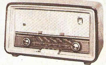
HORNYPHON Page S 1650.— Der besonders preiswerte UKW-Hochleistungs-Super mit Klangregister. Maße: 430 x 250 x 195 mm
