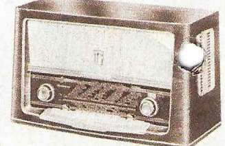
KAPSCH Univers S 2195.— Kraftvoller UKW-Luxussuper mit repräsentativer Ausstattung und hohem Bedienungskomfort. Duplex-Skalentrieb-automatik. Maße: 525 x 300 x 235 mm
