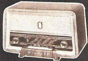
MINERVA Super-Minx S 1480.— Der bewährte 7-Röhren-UKW-Empfänger mit Klangregelung durch Drucktastenschaltung. Maße: 360 x 240 x 190 mm
