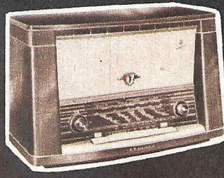
PHILIPS Pastorale S 3680. — Ein 10-Röhren-Luxussuper mit höchster Wiedergabetechnik und Klangqualität, transformatorlose Gegentaktendstufe. Maße: 675 x 445 x 315 mm
