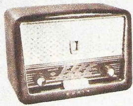
EUMIG Eumigette S 999.— Der UKW-Super mit dem verblüffenden Preis, 3 Drucktasten, Diskant- schalter für Baß- od. Höhenbetonung. Maße: 347 x 249 x 186 mm
