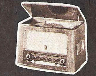
MINERVA Minerphon S 3520. — Ein UKW-Luxussuper, kombiniert mit 4-Geschwindigkeiten-Laufwerk, Duplex- antrieb, Ferritantenne. Maße: 590 x 410 x 360 mm
