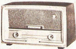
PHILIPS Rhapsodie S 1650.— Ein neuer PHILIPS-Empfänger mit Klangtasten, in modernem Gehäuse und mit geringem Preis. Maße: 430 x 250 x 195 mm
