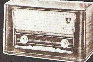
RADIONE Duplex Junior 58 S 1990.— Mehrpreis für 3D-Ausführung S 140.— Ein RADIONE-Mittelsuper mit der 2-Sender-Einstellung, drehbarer Ferritantenne, getrennter Baß- und Höhenregulierung und Klangregister. Maße: 514 x 292 x 215 mm
