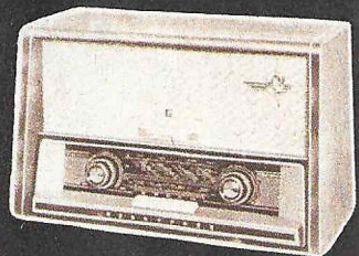
HORNYPHON Super-Prinz S 1898.— Dieser UKW-Fernsuper mit Klangregister, Ferroreceptor und „denkenden Tasten“ ist in seiner Preisklasse führend in Ton und Technik. Maße: 490 x 315 x 225 mm
