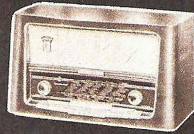
KAPSCH Sonocord S 1495.— Ein UKW-Vollsuper mit niedrigem Preis und der Leistung eines Großsupers, Klangregister. Maße: 444 x 260 x 210 mm
