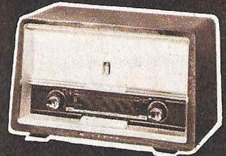
MINERVA Minercord S 1950. — Ein 7-Röhren-Super mit Drucktasten- bereichsschaltung, Drucktastenlang- register und Ferritantenne. Maße: 490 x 300 x 240 mm
