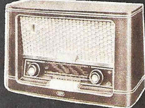
WSW-Tango 58 (SIEMENS) S 1780.— Mit Drucktasten und Klangregister, Bedienungskomfort durch fünf Drucktasten und getrennte Abstimmung des Mittel- und UKW-Bereichs. Maße: 470 x 295 x 204 mm
