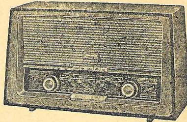
Page 7 Röhren, 430x250x195 mm, U-M- Wellen, Wechselstr. S 1650.—
