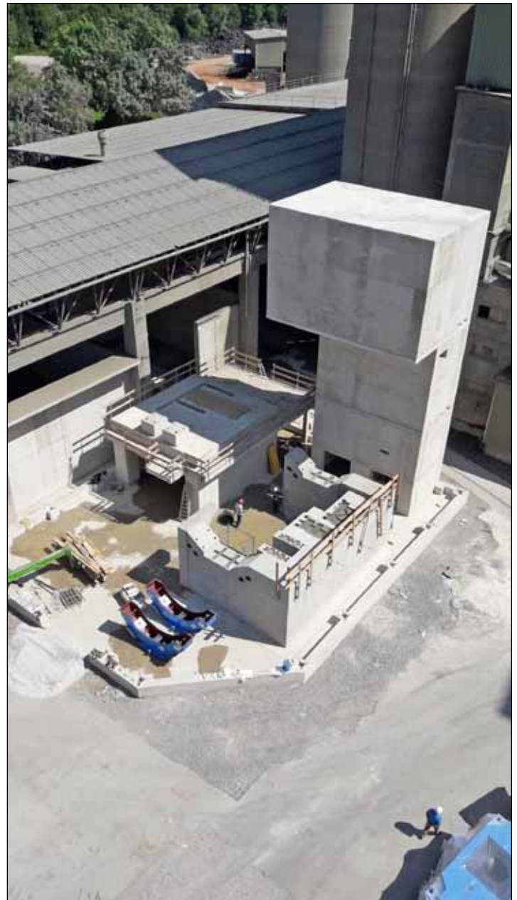
Fundamente und Elektroturm der neuen Zementmahanlage. Das Mühlengebäude wird in den nächsten Wochen fertiggestellt. (Foto: Schretter & Cie)
